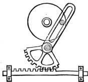
Fig. 23. CRANK-PIN.
