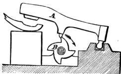
Fig. 21. WIPERS.
