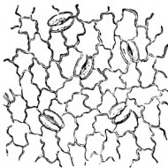
Fig. 1.—STOMATA.
